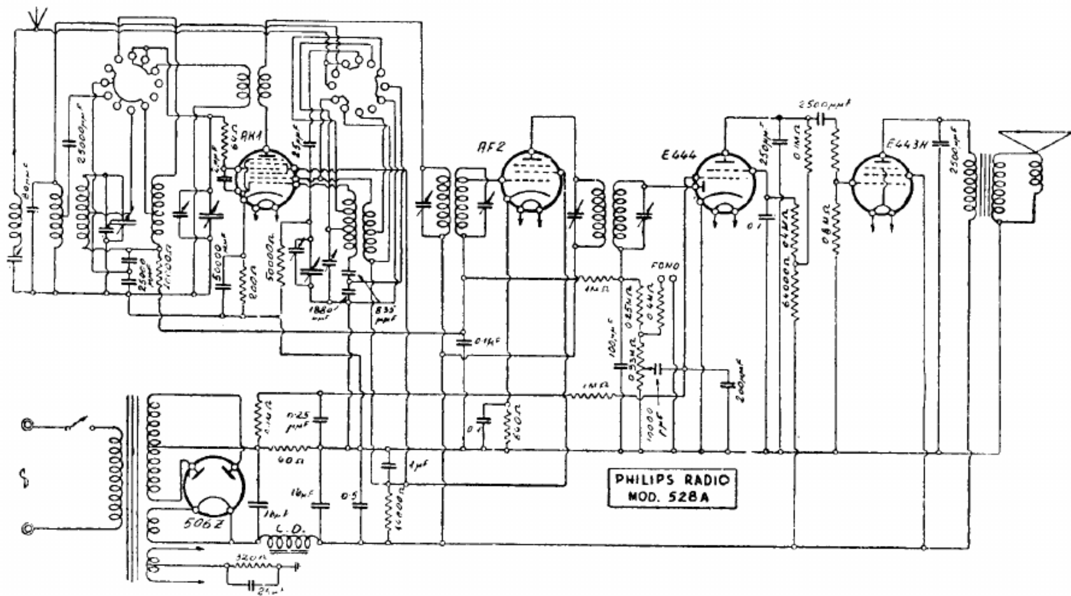
PHILIPS-RADIO — Modello « 528 A ». • Produzione 1935. Media frequenza: 125 kc.
